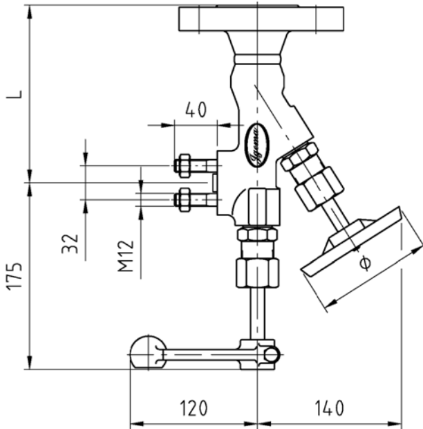
A210 with flange as per DIN
