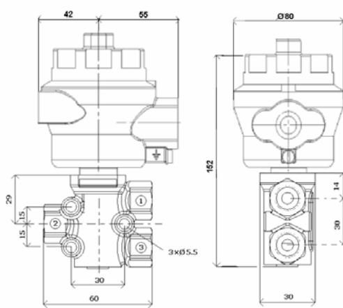
TYPE 309390 avec option capot anti-déflagrant ATEX : EExdIIC T6
