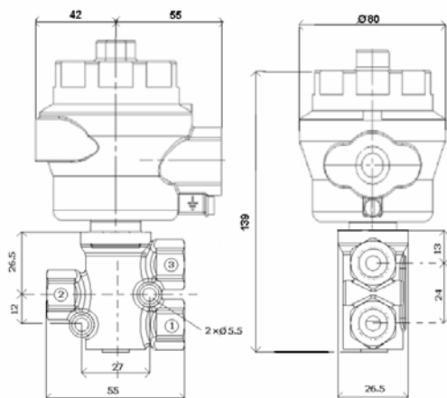
TYPE 306390 avec option capot anti-déflagrant ATEX : EExdIIC T6
